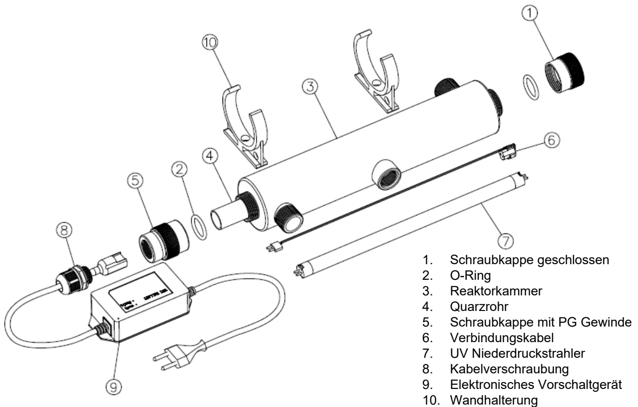
Abb.: Grundaufbau der UV-Anlagen mit einer Lampe
