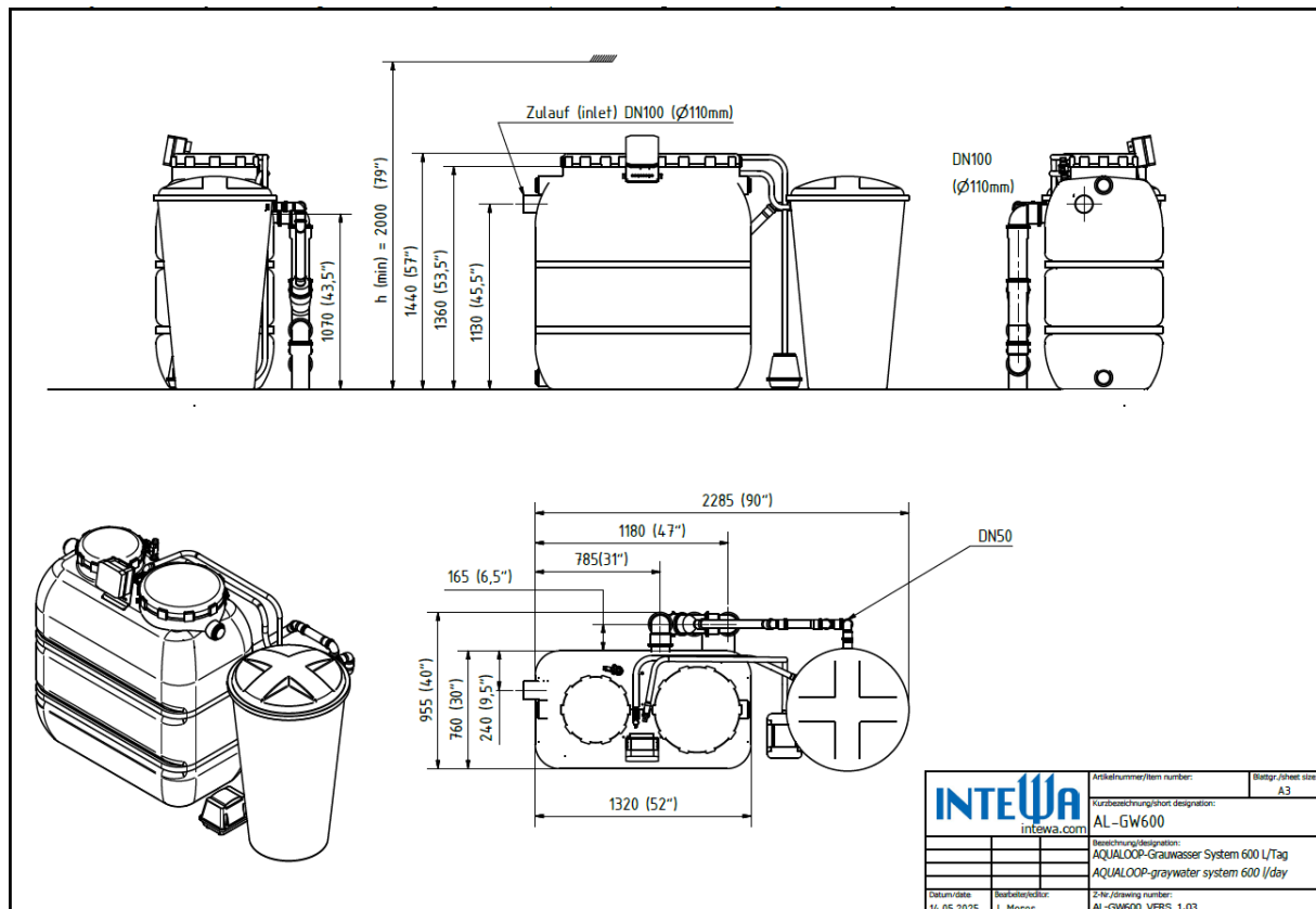
Figure 2 : Dimensions et connexions AQUALOOP AL-GW600 l/d
