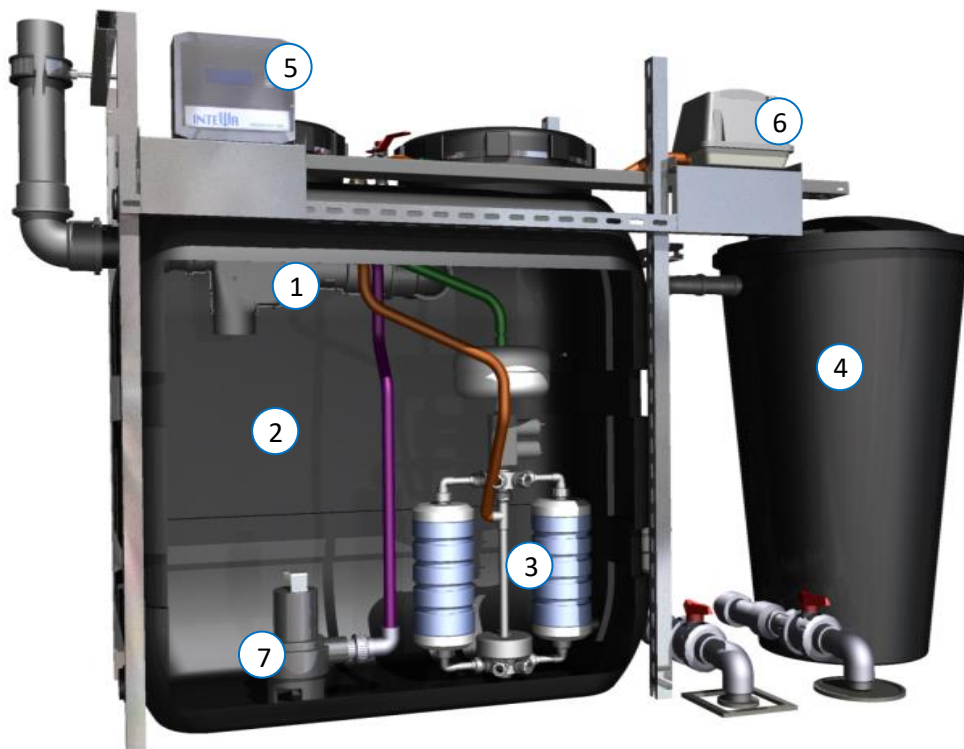
Figure 1 : Vue d'ensemble : Système emballé AQUALOO Système de recyclage des eaux grises 600 l/jour
