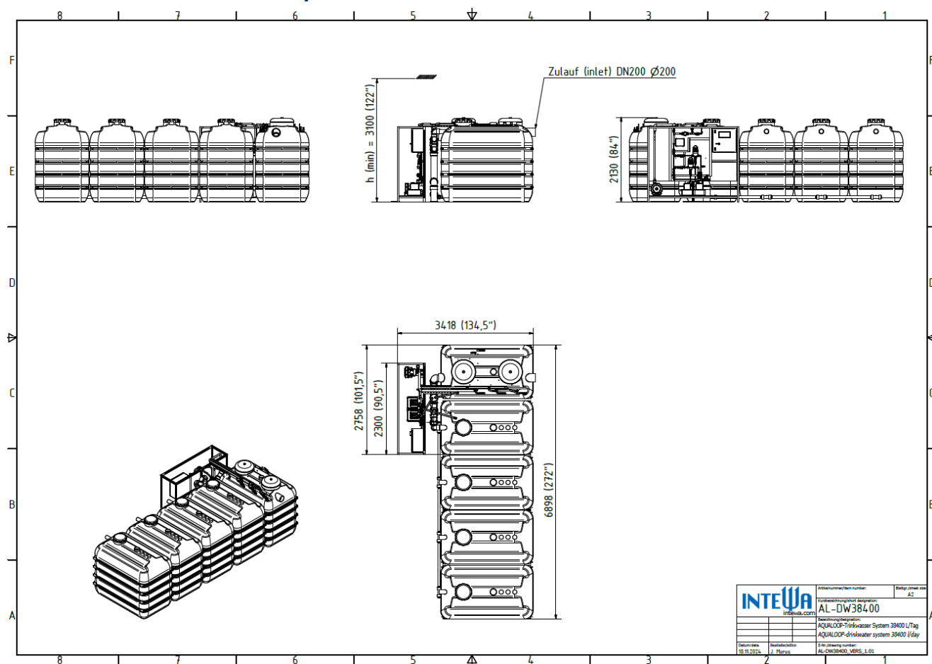
Figure 2 : Dimensions et connexions AQUALOOP AL-DW38400 I/d
