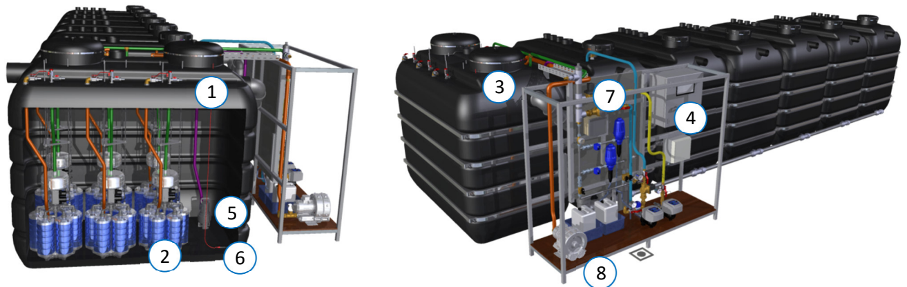
Figure 1 : Vue d'ensemble : Système emballé AQUALOOP Système d'eau potable 57600 l/jour
