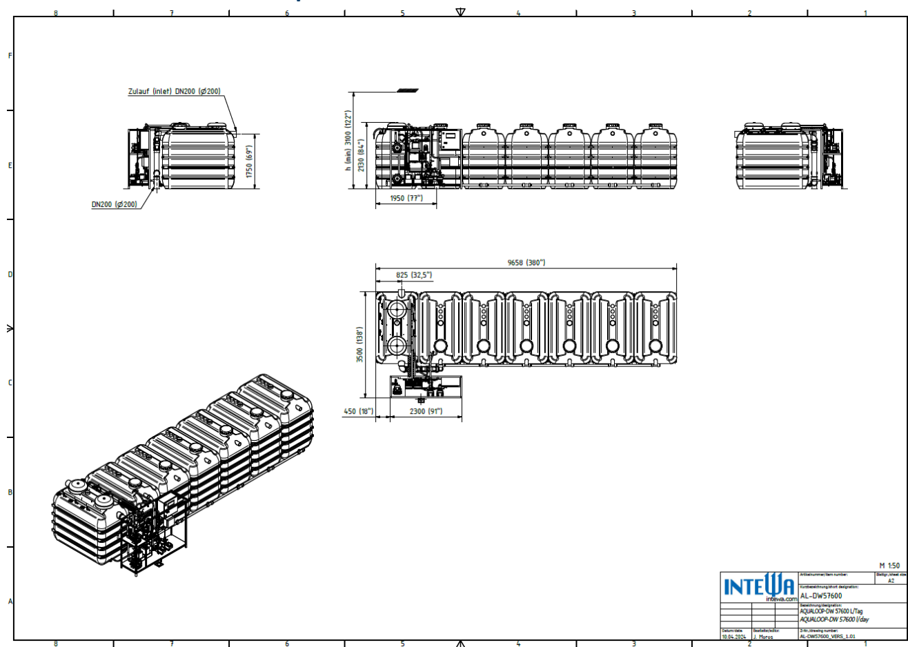
Figure 2 : Dimensions et connexions AQUALOOP AL-DW57600 I/d
