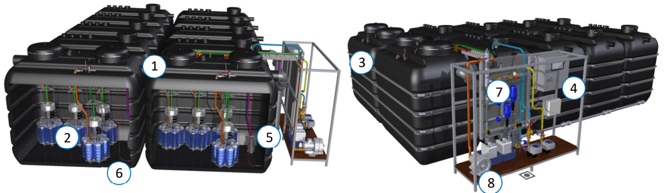
Figure 1 : Vue d'ensemble : Système conditionné AQUALOOP Système d'eau potable 86400 l/jour
